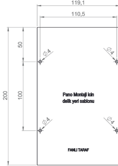
Şekil 7: Statik Kontaktör Mekanik Bağlantı Şablonu
